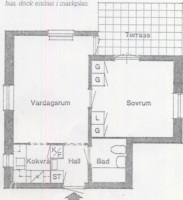
2 rum och kokvrå ca 43 m 2 .
